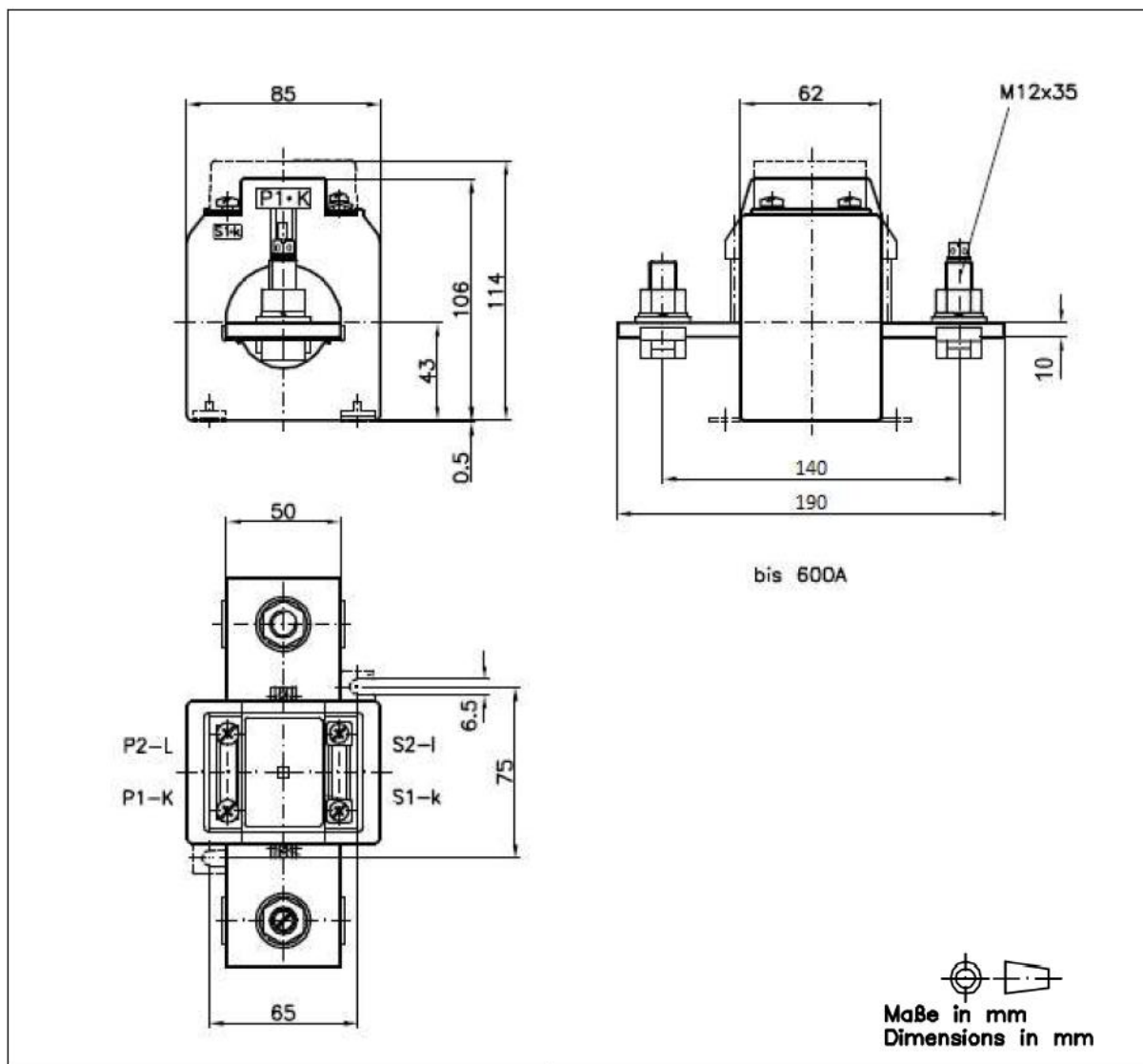
Abbildung 9 - Stromwandler
