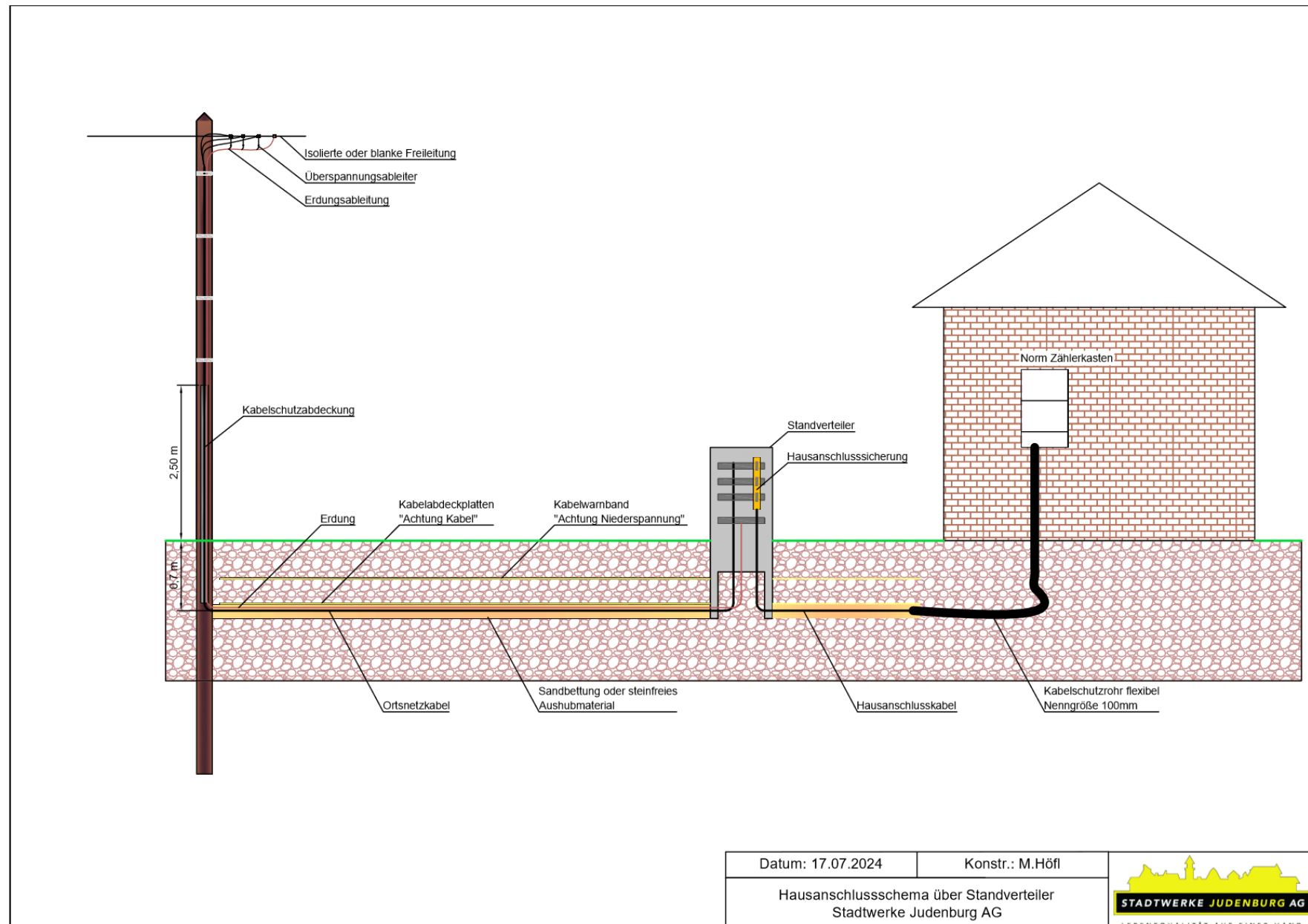
Feb 26 Abbildung 1: Hausanschlussschema über Standverteiler
