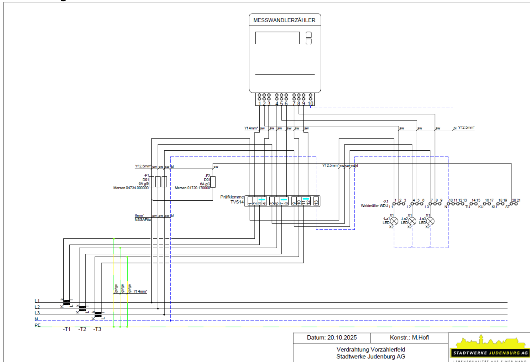
Abbildung 11 - Verdrahtung Vorzählerfeld
